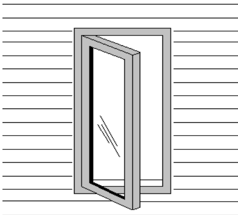
Fenêtre à battant gauche / Casement left handed
